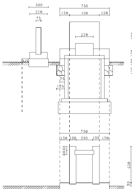
ア 正面図
