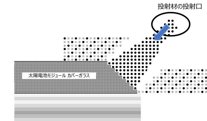
図表 40 ブラスト工法
