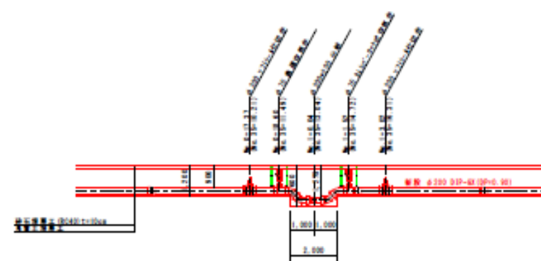
分岐部配管断面図 S=1:100 原設計どおり
