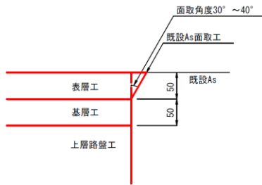
既設As面取工断面図 S = 1 : 5
