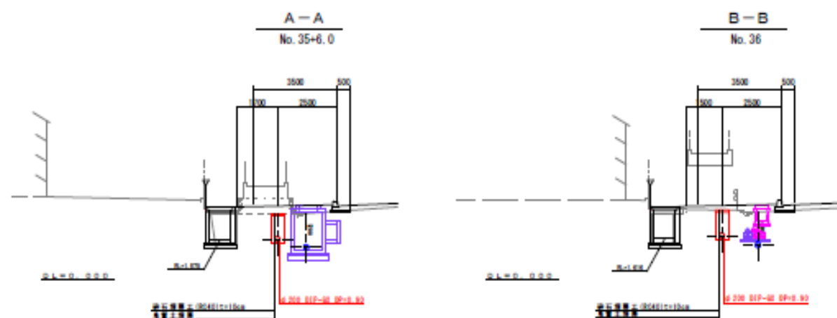
横断図 S=1:100 原設計どおり
