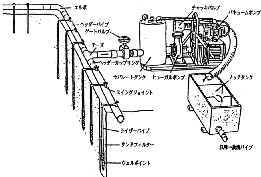
図 1-1 ウェルポイントポンプ設置標準図
