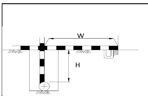
布設位置
