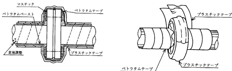
図1 絶縁フランジ部の処理
