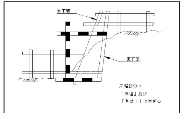
切取り法面
