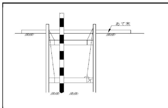
腹起し切梁の設置間隔
