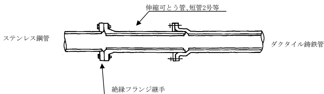
図2 異種金属管の接続 (ダクタイル鋳鉄管とステンレス鋼管との接続法)
