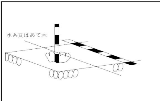
碎石基礎工(転圧完了後)
