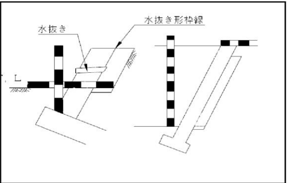
石 積
