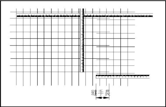
各部配筋寸法
