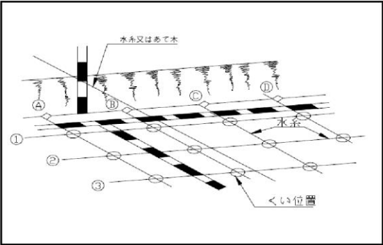
施工前くい位置
