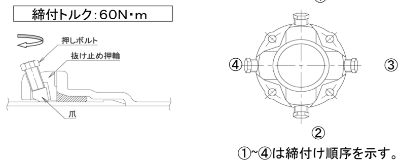
図-3.11 押しボルトの締め付け
