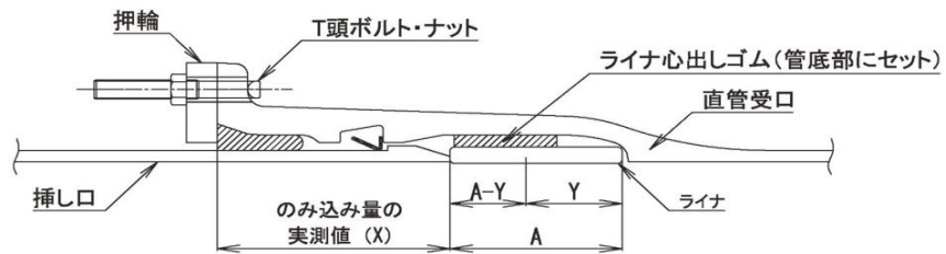
図-3.14 ライナ使用時の接合構造図
