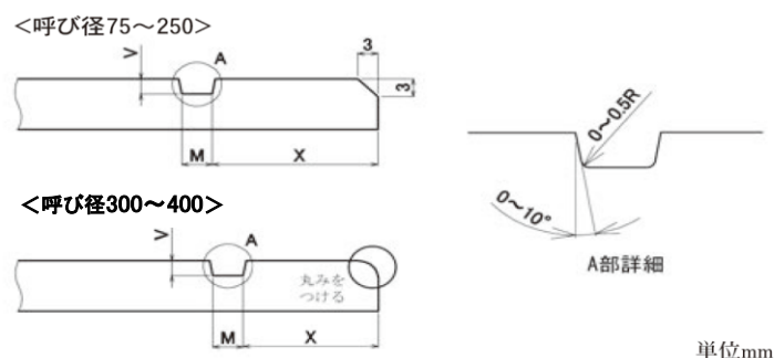
図-3.2 挿し口加工寸法
