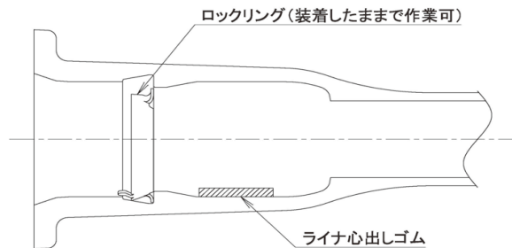
図-3.12 ライナ心出しゴムのセット
