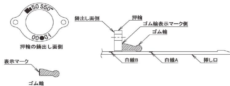
図－3.7 接合部品のセット位置
