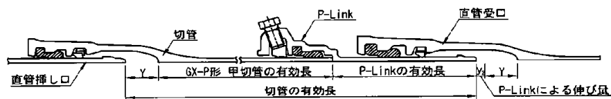
図-3.1 P-Linkを用いた切管有効長
